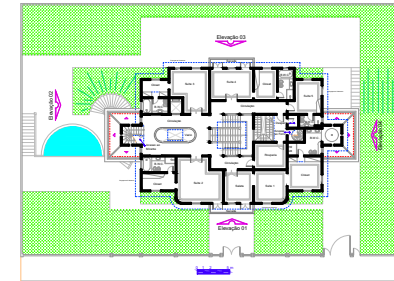
Superior A = 330,41 m 2
