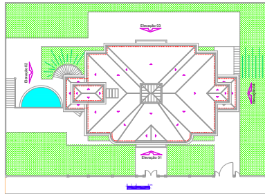
Implantação e Cobertura
