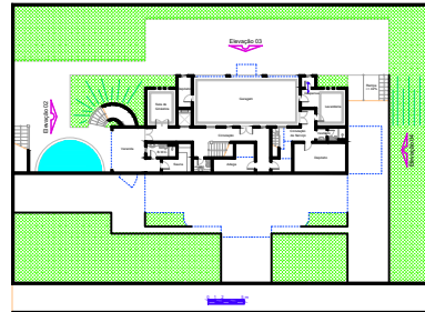
Subsolo A = 239,66 m 2
