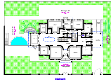
Térreo A = 367,76 m 2
